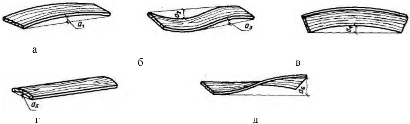
Рисунок 46 –Измерение покоробленности
