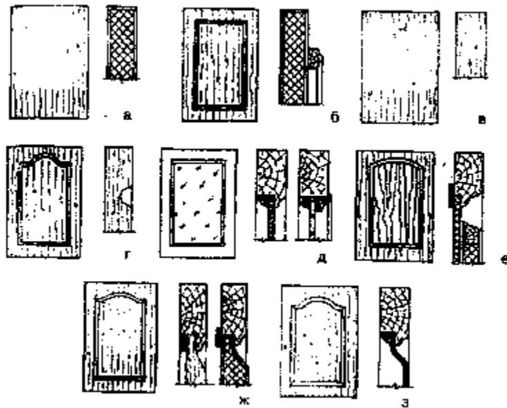
Рисунок 26- Конструктивные решения дверей
