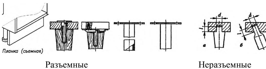
Рисунок 33 – Виды подсадных ножек
