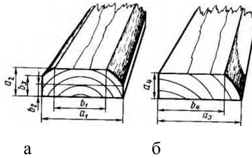
Рисунок 45 – Измерение обзола
