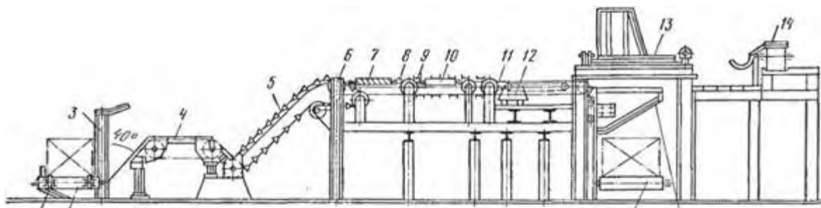
Рисунок 57 - Пакетоформирующая машина ПФМ-10
