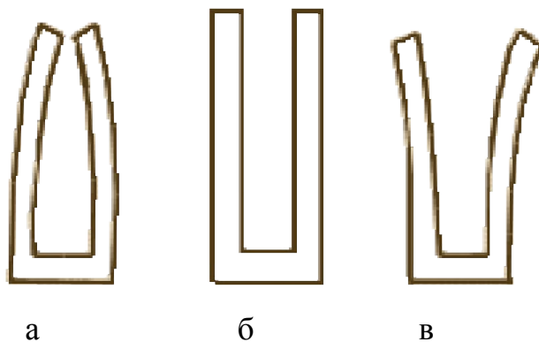
Рисунок 60 – Возможные деформации силовой секции
