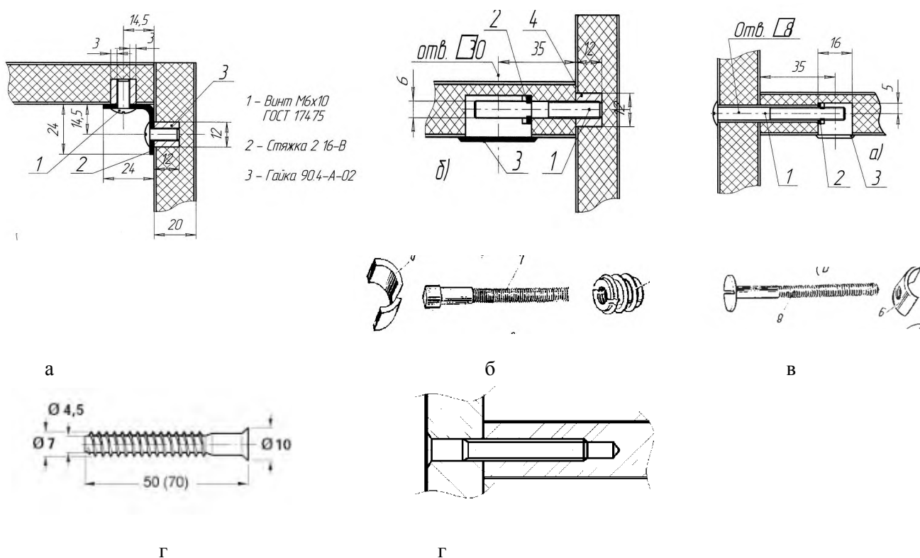
Рисунок 25 - Виды стяжек
